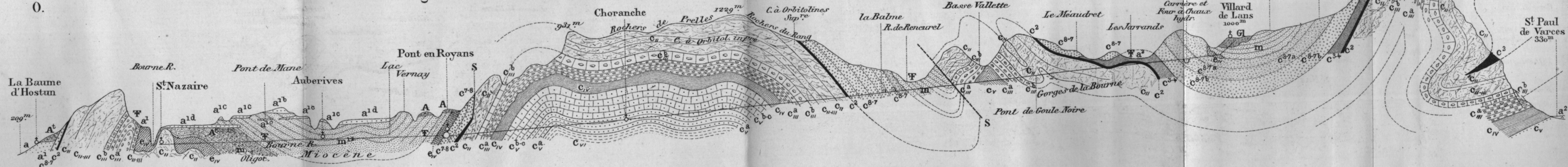
Fig. 4 — Coupe de la Baume d'Hostun à St. Paul de Varcès le long de la Vallée de la Bourne, par W. Kilian (Echelle des hauteurs triple de celle des longueurs).
