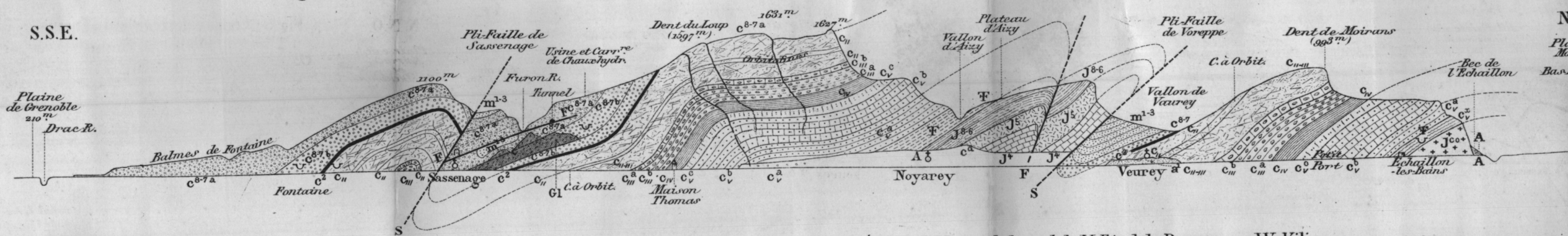
Fig. 4 — Coupe de la Baume d'Hostun à St. Paul de Varcès le long de la Vallée de la Bourne, par W. Kilian (Echelle des hauteurs triple de celle des longueurs).
