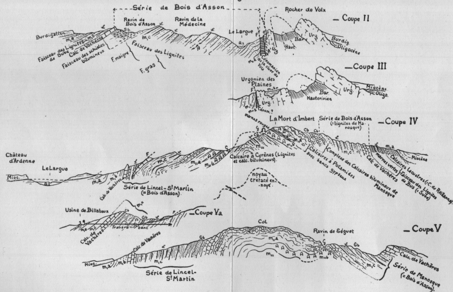
PLANCHE II. — Série de coupes géologiques de l'anticlinal de Volx. La position de ces coupes est indiquée sur la carte géologique planche I.
