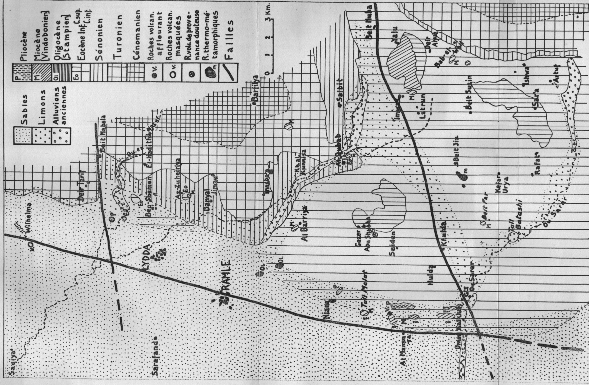
CARTE GÉOLOGIQUE DE LA RÉGION ARTUF-LYDDA
