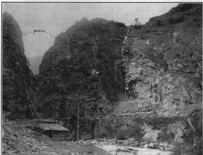
PL. III-B. — APPUIS DU BARRAGE AU VERROU DU CHAMBON.
