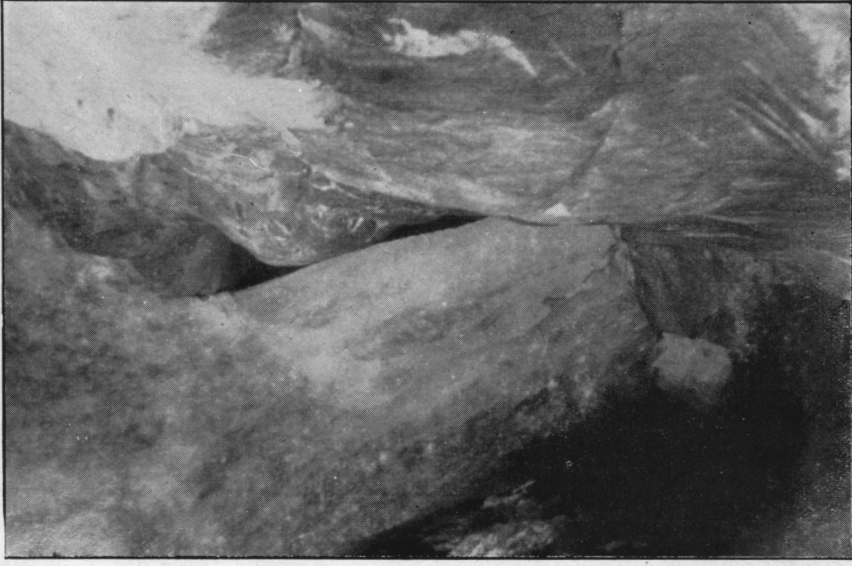
Pl. IX B. — Stries glaciaires sur un rocher de la rive gauche vu de l'amont; grotte sous-glaciaire.
