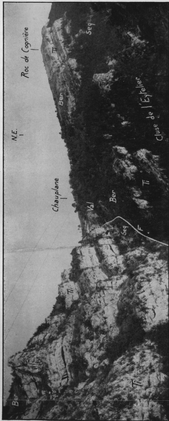
LA FAILLE DE CHAUPLANE (vue de la route de la Bâtie à St-Michel-les-Portes). ( Val , marnes valanginiennes; Ber , Berriasien; Ti , Tithonien et Kimméridgien; Séq , Séquanien; F , faille de Chauplane).
