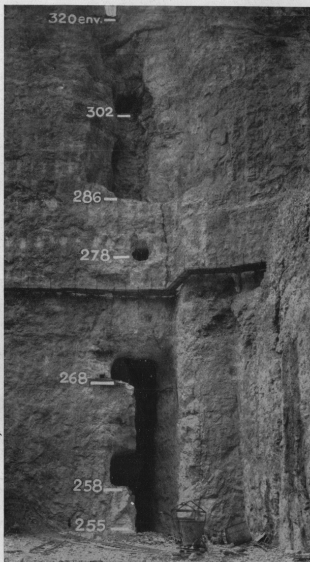
PL. IV. — Aven fossile (éocène) découvert dans l'Urgonien de la rive droite à Génissiat.
