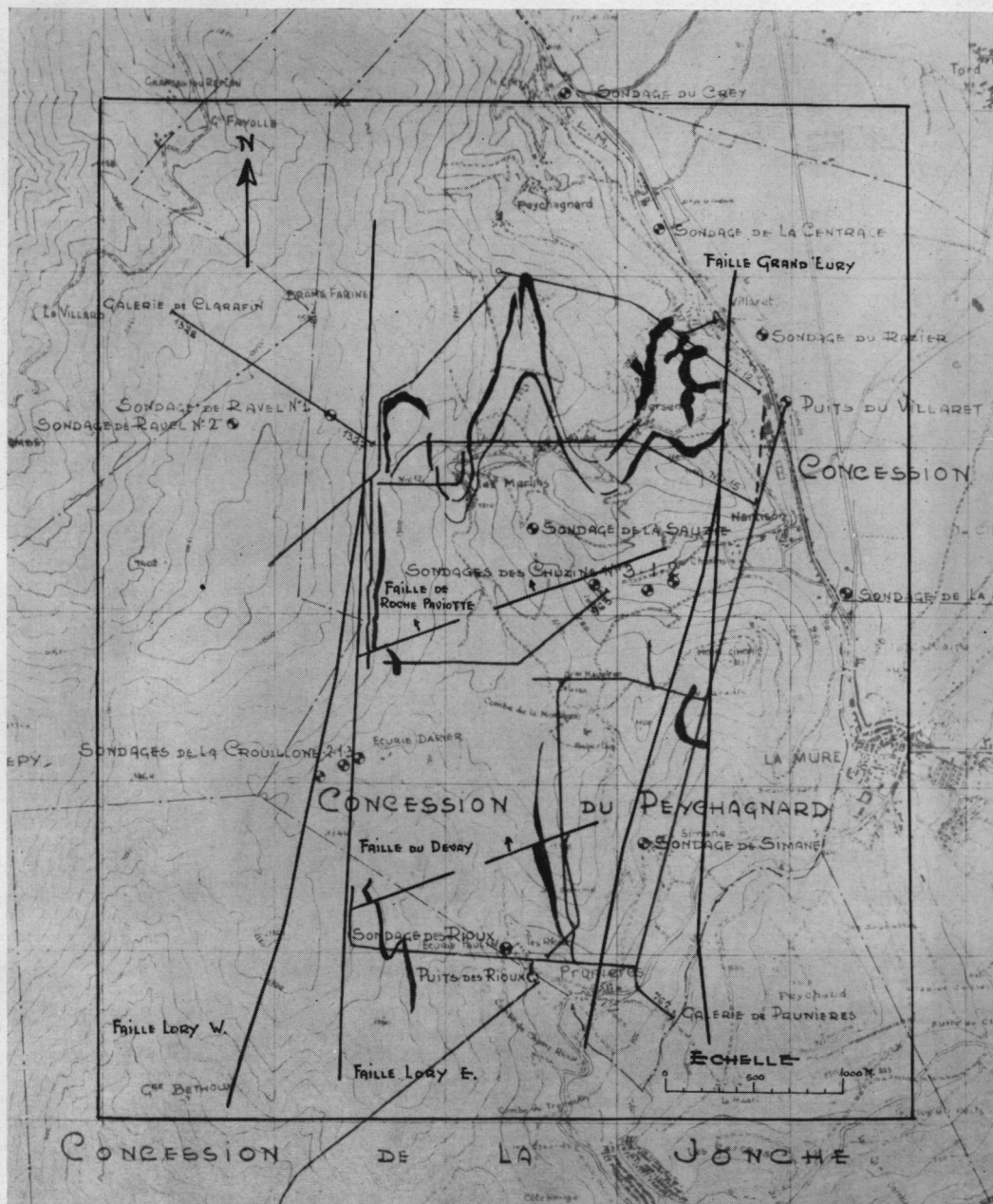
Fig. 1. — Plan d'ensemble des exploitations des Houillères du Bassin du Dauphiné. Le dédoublement Ouest de la faille Grand'Eury a été observé au fond et n'a pas encore été vu en surface.
