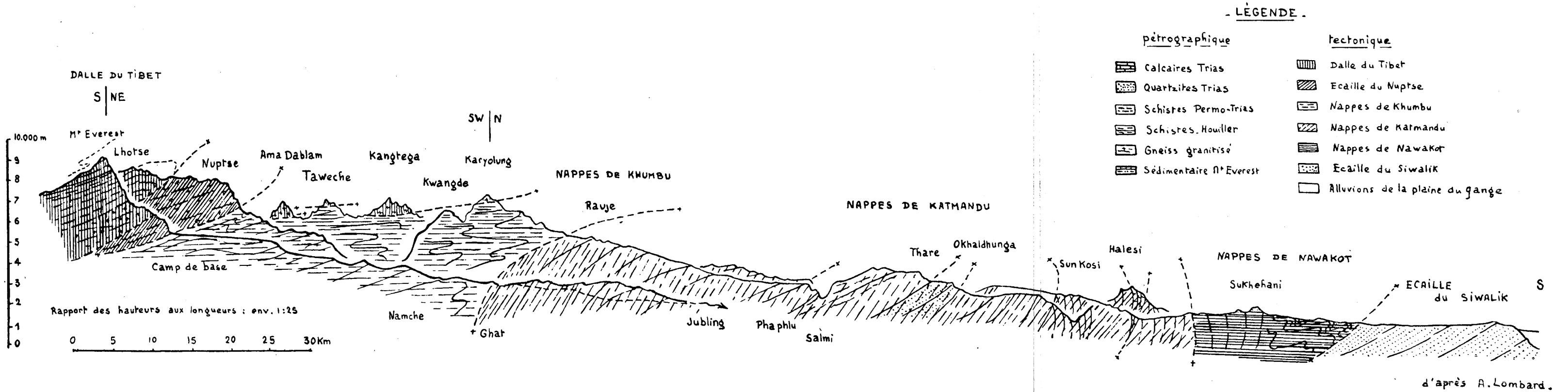
Coupe 5
