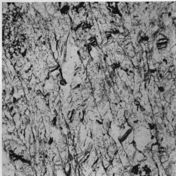
Fig. 1. — Grès Permien. Collet d'Allevard.
