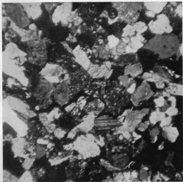
Fig. 2. — Grès Permien. Le Luc Provence.
