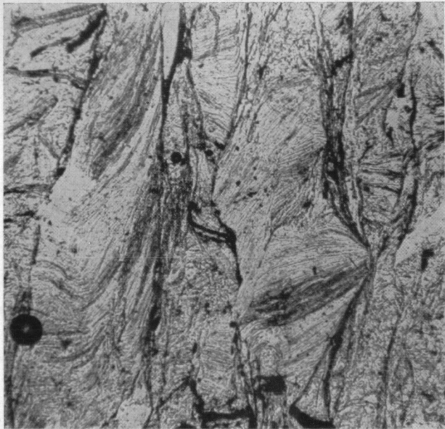
Fig. 1. — Grès Permien. Pré de l'Arc.
