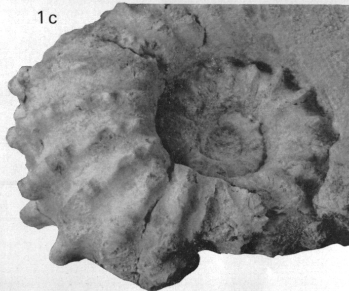
Fig. 1. — Douvilleiceras leightonense pringlei Casey, route de Coulmes (Isère). 1a : vue ventrale du stade évolué; 1b : détail du flanc gauche du dernier tour; 1c : vue oblique de la tuberculation juvénile; \times 1 .
