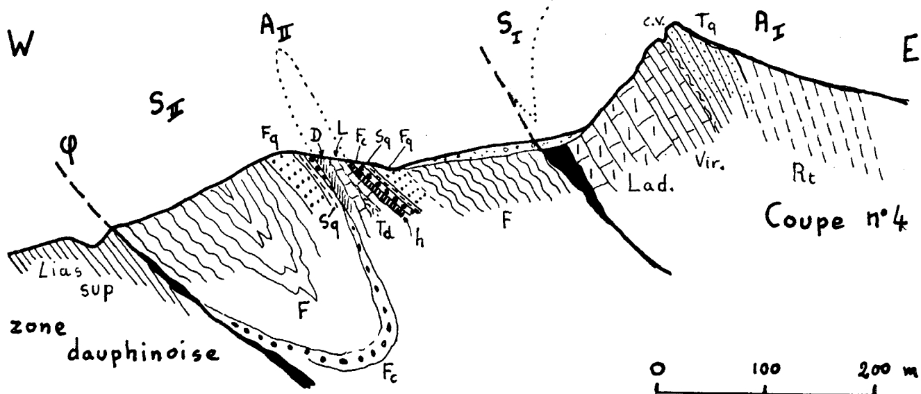
Fig. 4. — Coupes dans la zone des plis isoclinaux externes.
