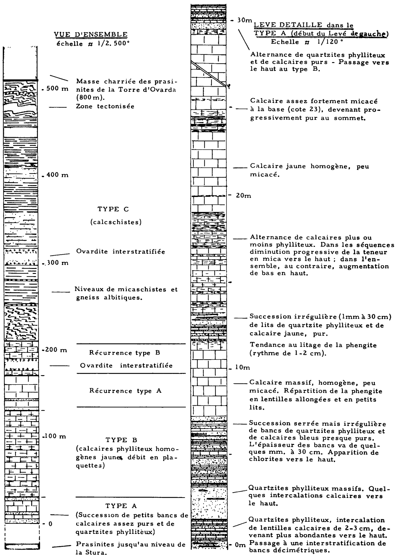
Fig. 2. — Levés détaillés dans la série des Schistes lustrés, au-dessus d'Usseglio — A gauche : vue d'ensemble. — A droite : levé détaillé dans le faciès de base (type A).
