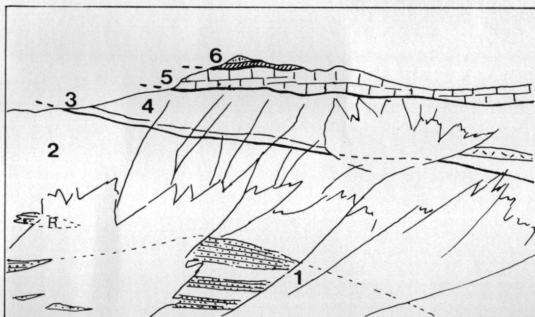
PL. IX. — CONTACT DES NAPPES DE L'EMBRUNAIS-UBAYE SUR L'AUTOCHTONE AU SE DE DOURMILLOUSE.
