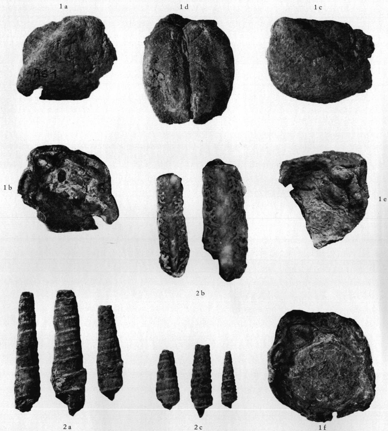
Fig. 1. — Epicyprina lamartrensis nov. sp. Holotypes. X 1. Valanginien de La Martre (Var). Coll. I. G. A. L., Paris. 1 a : Valve droite ; 1 b : Charnière de la valve droite ; 1 c : Valve gauche ; 1 d : Valves en connexion ; 1 e : Charnière de la valve gauche ; 1 f : Une valve droite montrant la charnière (la dent 3 b est incomplète).
