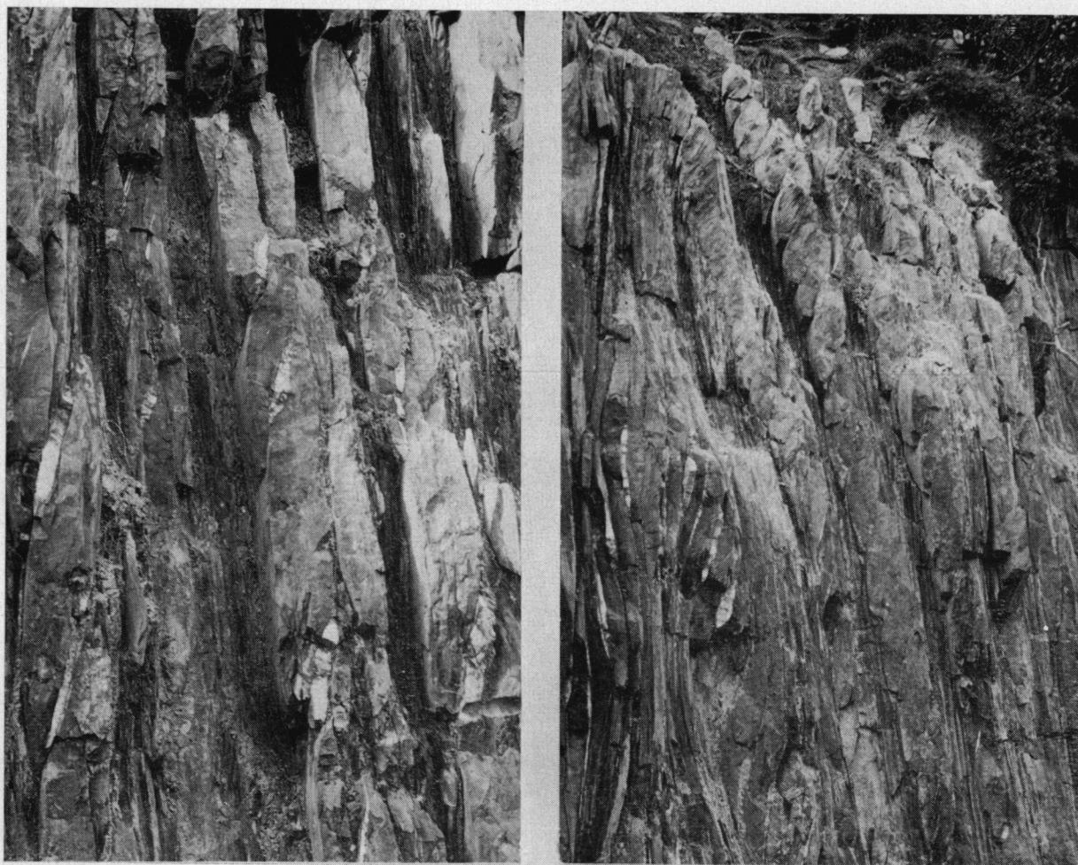
Fig. 1. — Microlithons sur le flanc oriental d'un anticlinal N-S. Vue en direction du N.
