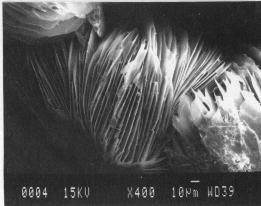
Figure 2 : Feuilletes de cookéite vus à un plus fort grossissement (x400)
