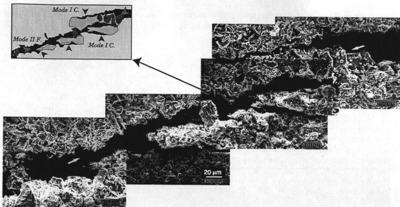
FIG. 2. – Coalescence des fractures de mode I et développement des fractures de mode II.
